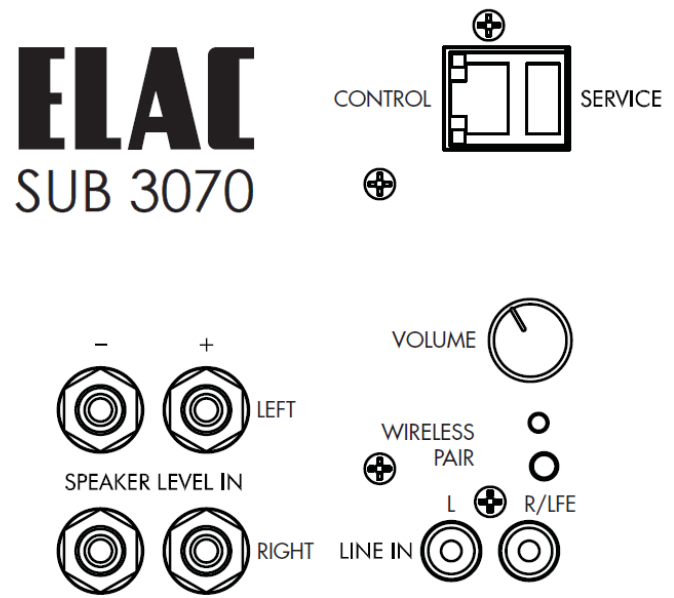
Bouton de jumelage sans fil caisson d'extrêmes basses SUB3070
