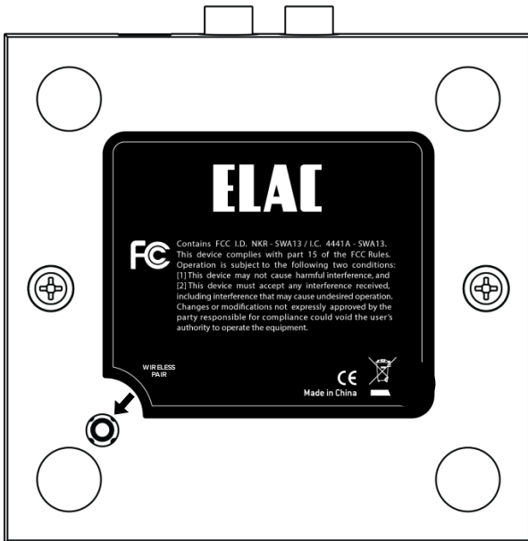
Bouton de jumelage sans fil AirX 2
