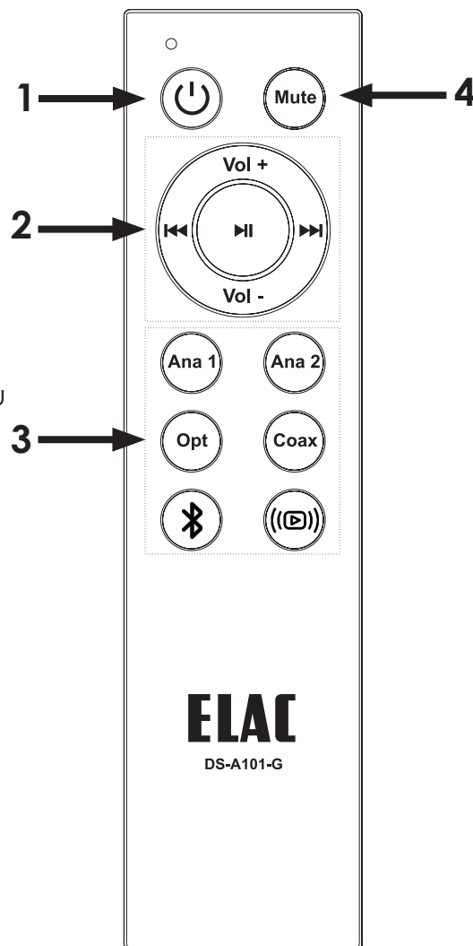
Figure 3 Fonctions de la télécommande infrarouge DS-A101-G
